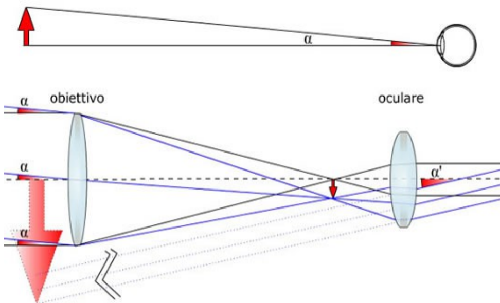
Schema ottico del cannocchiale di Keplero
